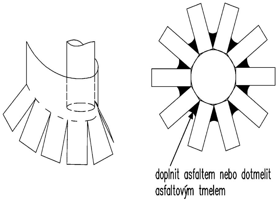
Obrázek /33/ – Princip kalhotek
