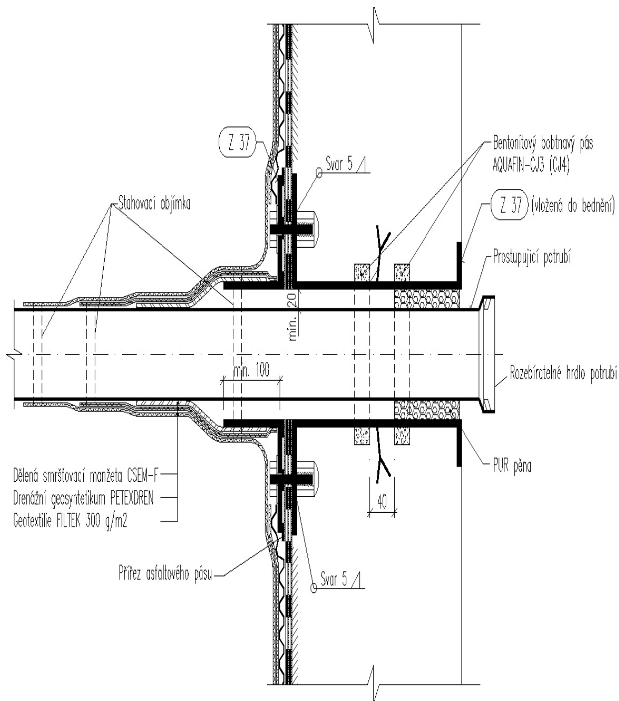
Obrázek /36/ Příklad řešení prostupu asfaltovými pásy s použitím příruby
