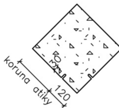
Koutová tvarovka 3 (s posypem)
