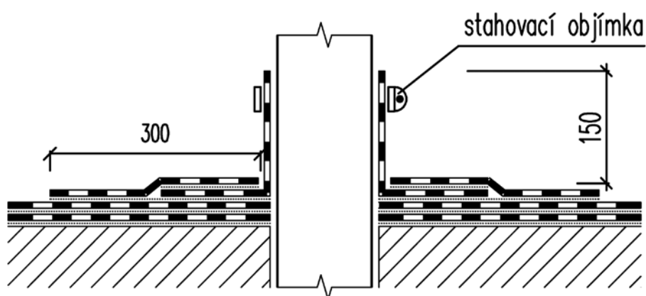
Obrázek /31/ Schéma opracování detailu kruhového prostupu
