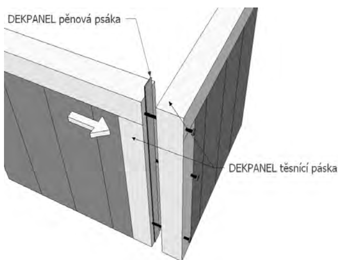
Schéma 5: Rohové spojení panelů kolmo umístěnými vruty
