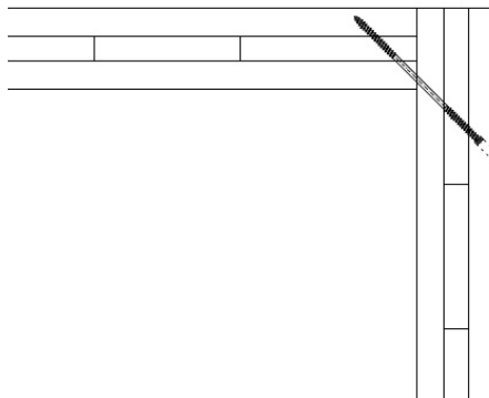
Schéma 4: Vruty šroubované horizontálně pod úhlem 45°
