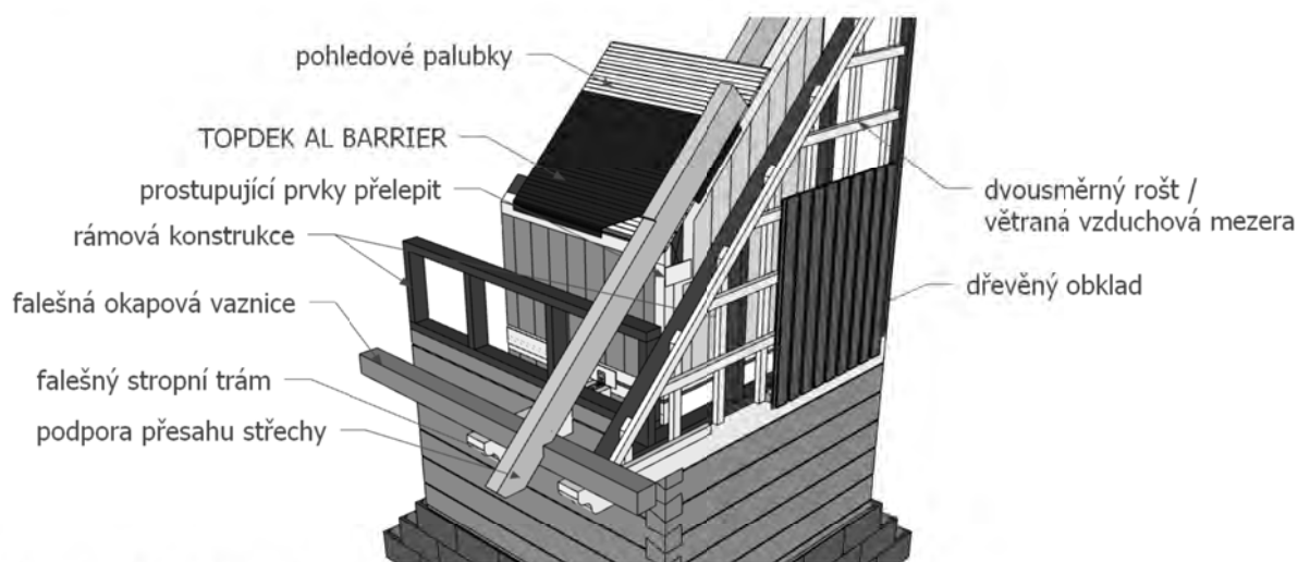
Schéma 20: Ná vaznosti okapní a štítové hrany
