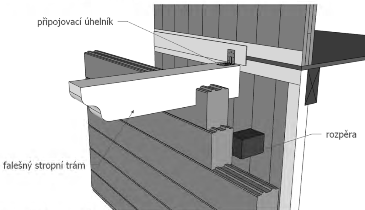
Schéma 18: Osazení falešných stropních trámů
