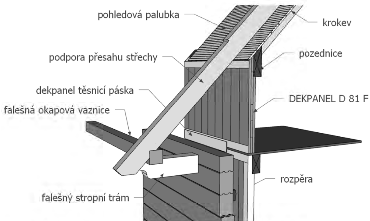
Schéma 19: Řešení okapní hrany – rozpracovaná tesařská konstrukce
