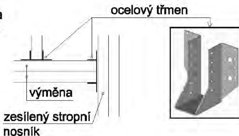
Schéma 10: Řešení prostupů stropní konstrukcí
