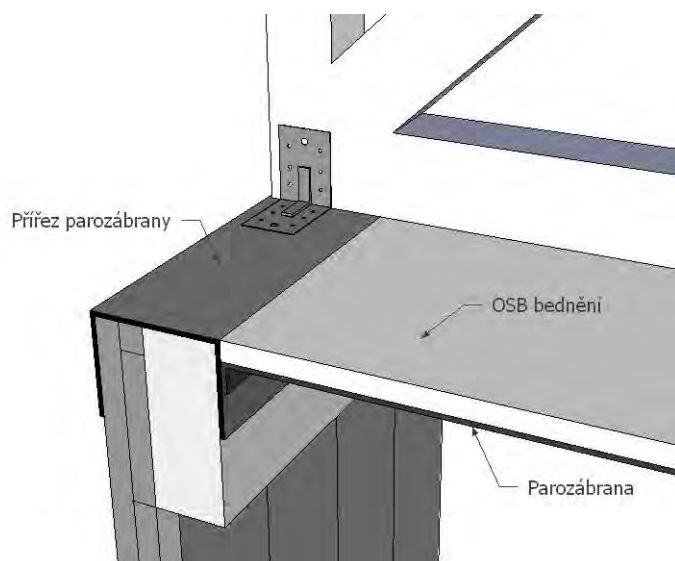
Schéma 14: Uložení příhradových vazníků - bez stropní konstrukce
