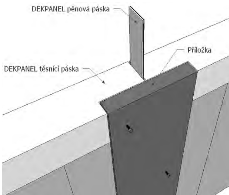
Schéma 3: Průběžné propojení panelů
