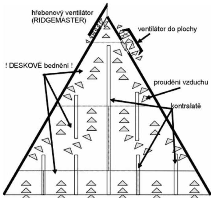
Obr 8.4. Schéma odvětrání stanové či podobné střechy
