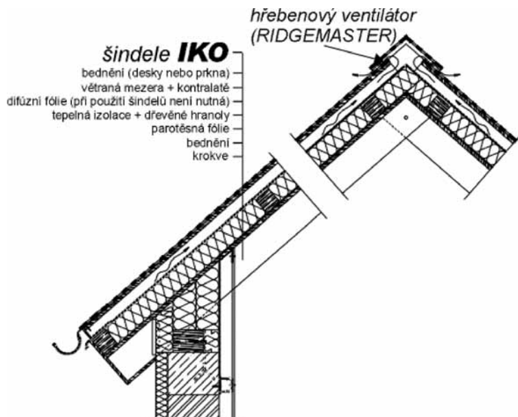
Obr 8.4. Schéma odvětrání stanové či podobné střechy
