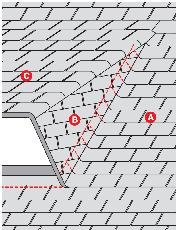
Obr. 7.1. Víkřové okno s nízkým sklonem a strmými postranními stranami
