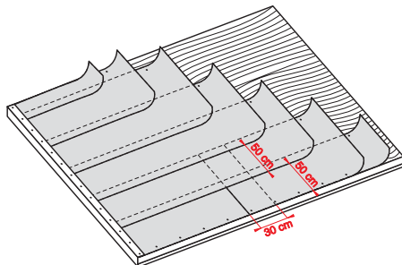
Obr. 3.2. Dvojnásobný přesah podkladního pásu u nízkých sklonů střechy (15° - 20°)
