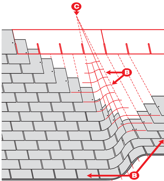
Obr. 7.2. Vířivé okno se strmým sklonem střechy a malými zaoblenými bočními stranami
