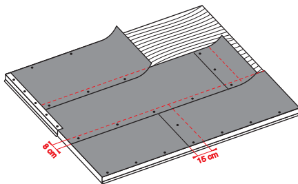
Obr. 3.1. Pokládka speciálního samolepivého pásu Armourgard Ice & Water Protector® u nízkých sklonů střechy
