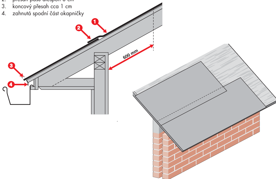
Obr. 3.4. Ochrana příokapní části střechy pásem Armourgard Ice & Water Protector®
