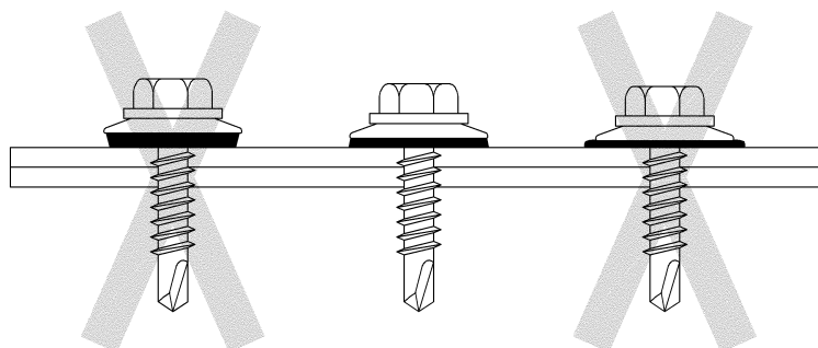
Obr. 9: Dotahování šroubů
