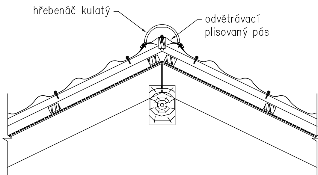
Obr. 16: Nároží
