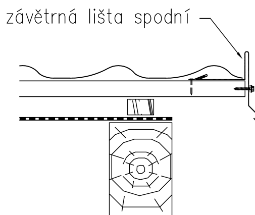
Obr. 11: Závětrná lišta spodní
