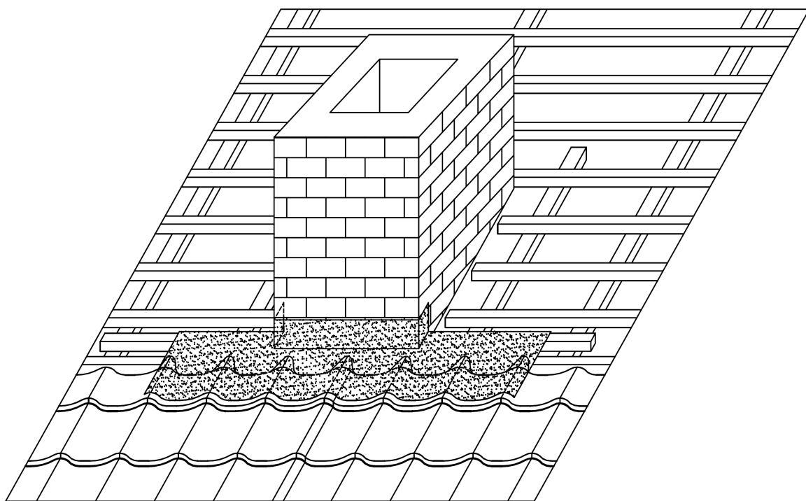
Obr. 17: Osazení plisovaného pásu a vytvarování
