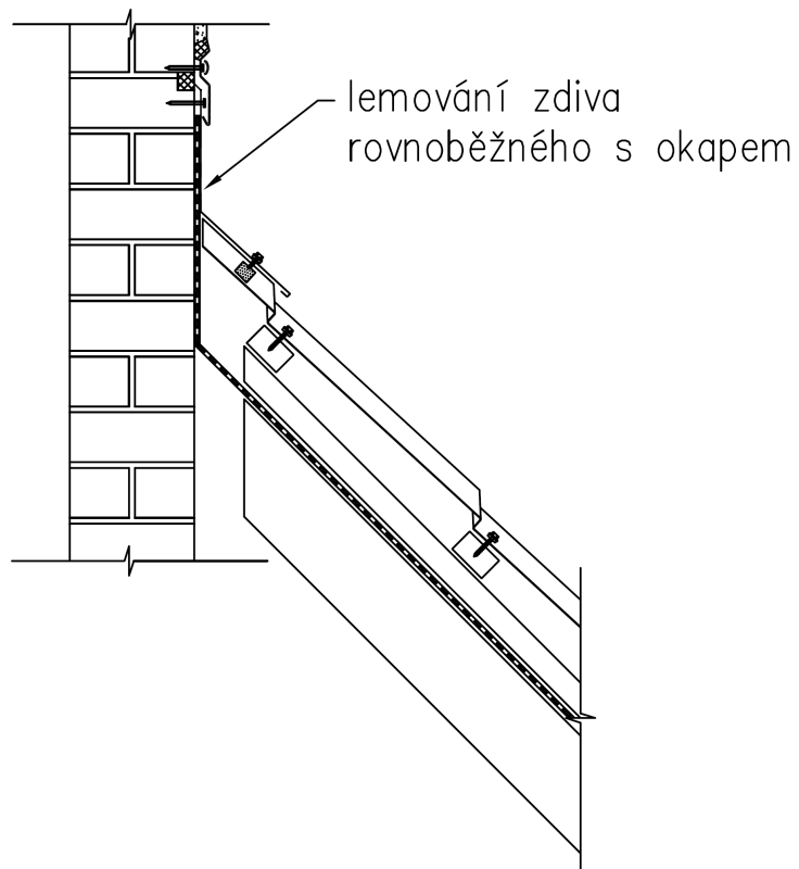
Obr. 24: Ukončení krytiny u stěny rovnoběžné s okapem
