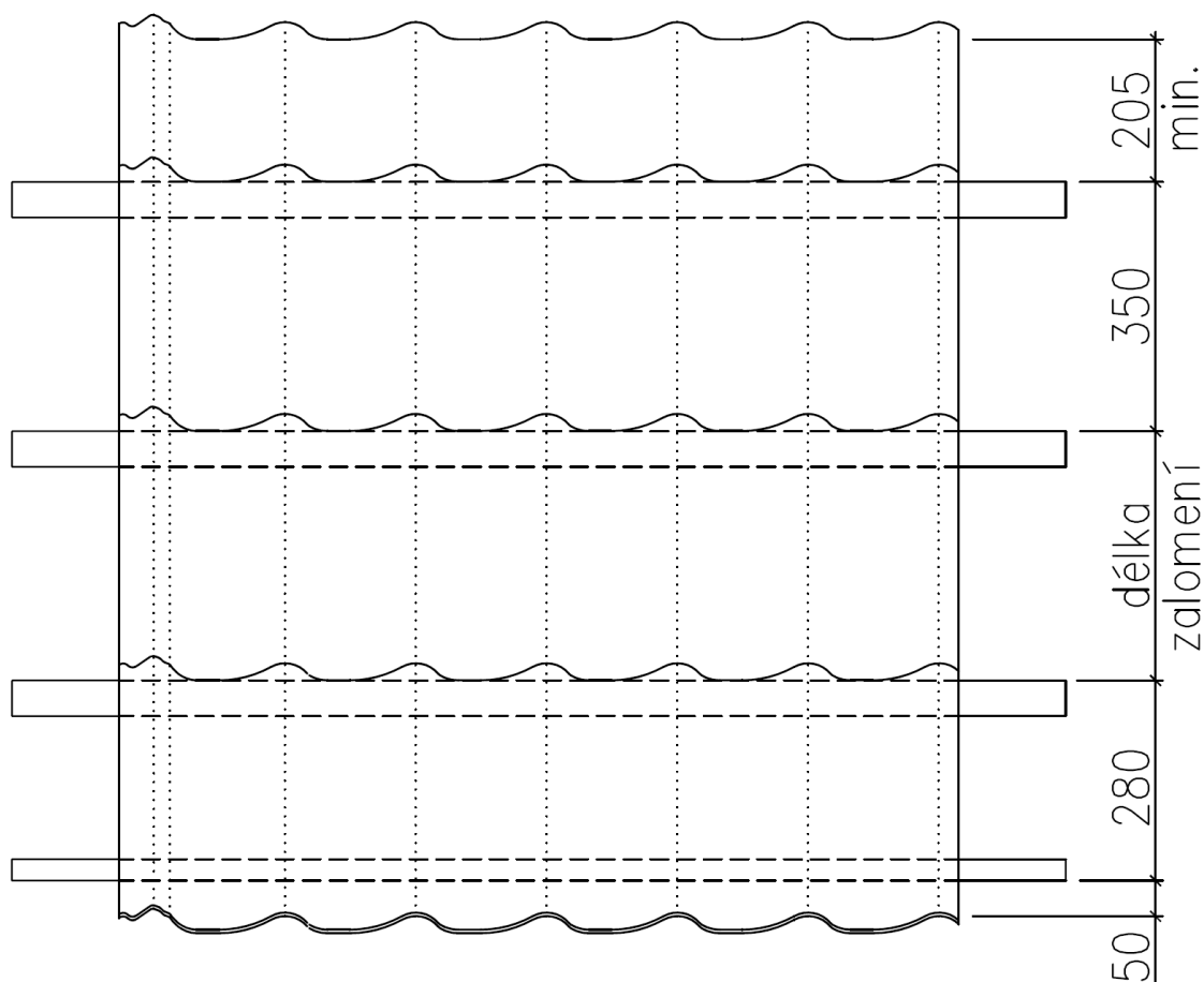
Obr. 5a: Rozměření latí pro krytí
