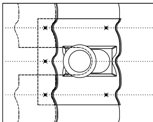
Obr. 28b: Osazení vrchní tabule
