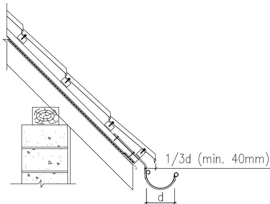
Obr. 10: Okap
