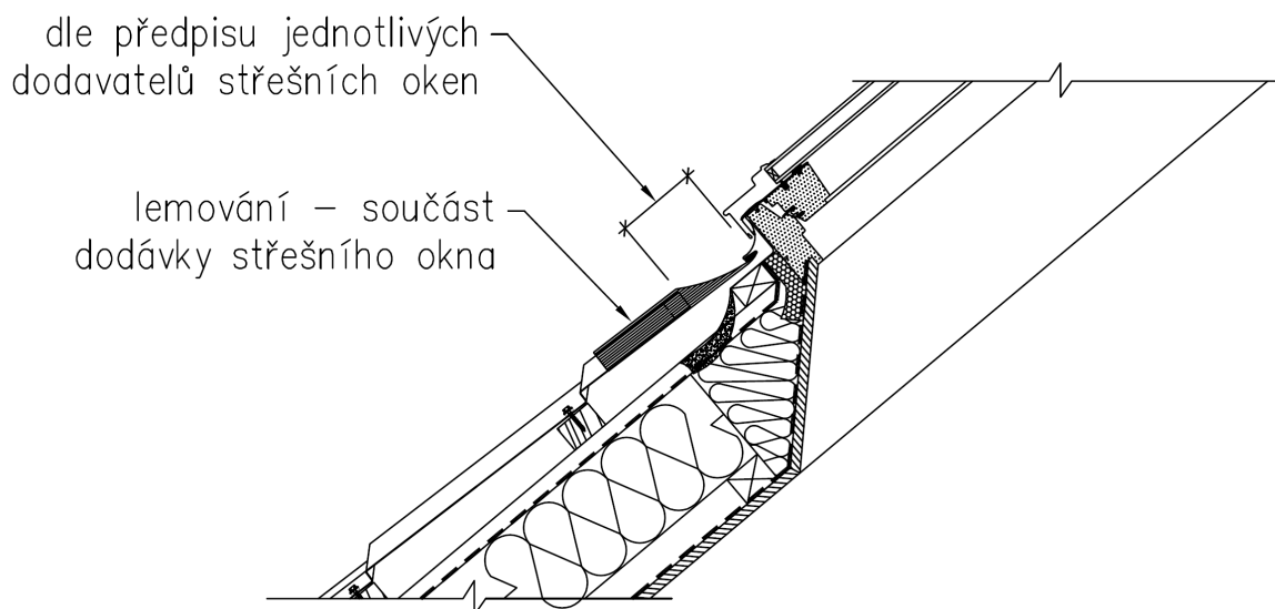
Obr. 26: Spodní napojení střešního okna
