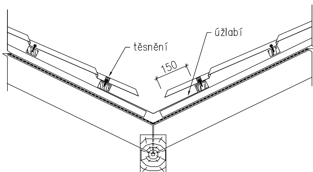
Obr. 15: Úžlabí
