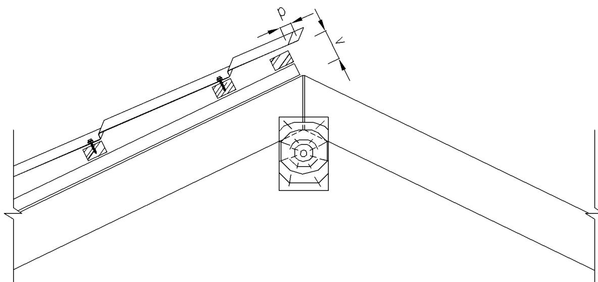
Obr. 4: Prodloužení krytiny oproti délce krokví u hřebene
