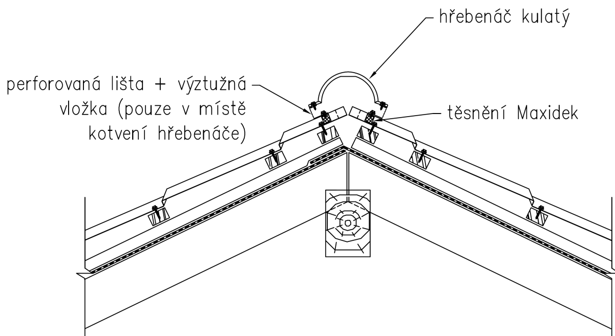
Obr. 13: Větráný hřeben
