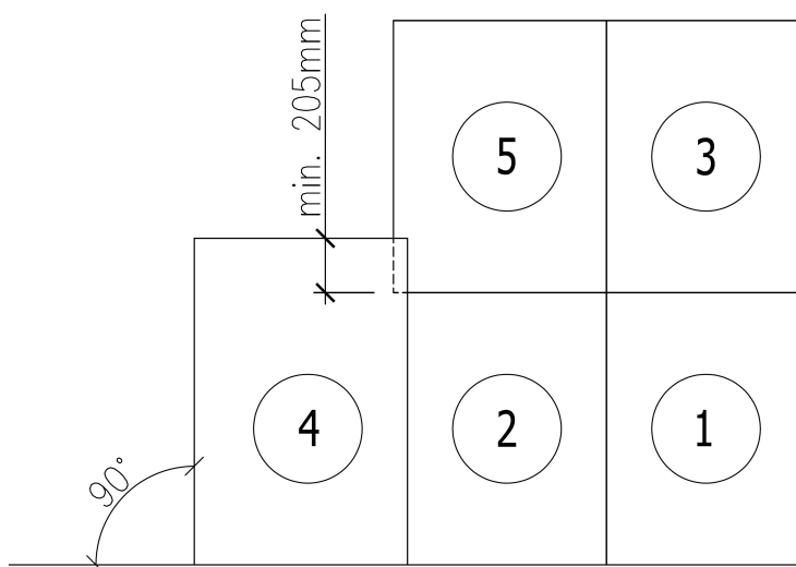
Obr. 6: Pořadí kladení jednotlivých tabulí
