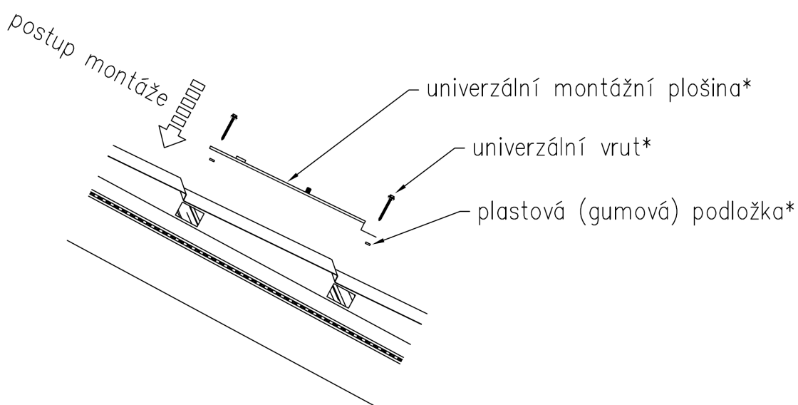
Obr. 29: Osazení univerzální montážní plošiny
