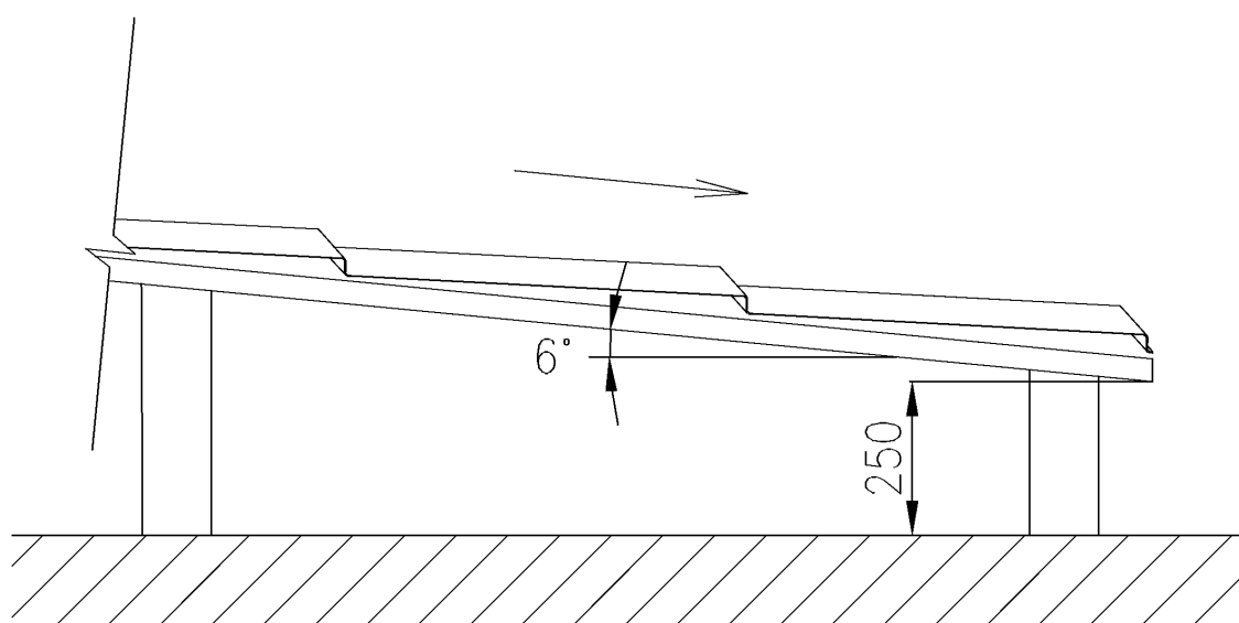
Obr. 3: Schéma skladování krytiny
