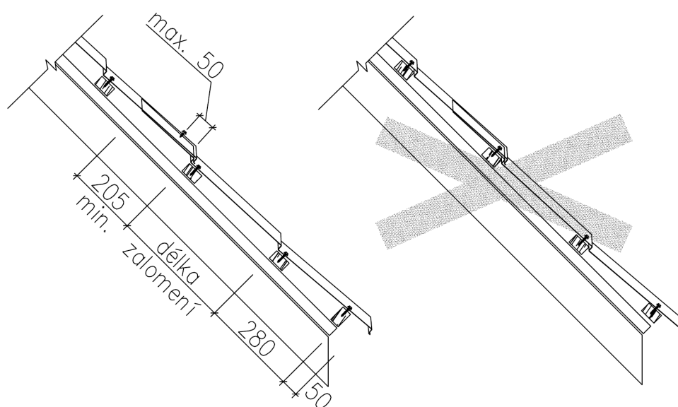
Obr. 5b: Rozměření latí pro krytí
