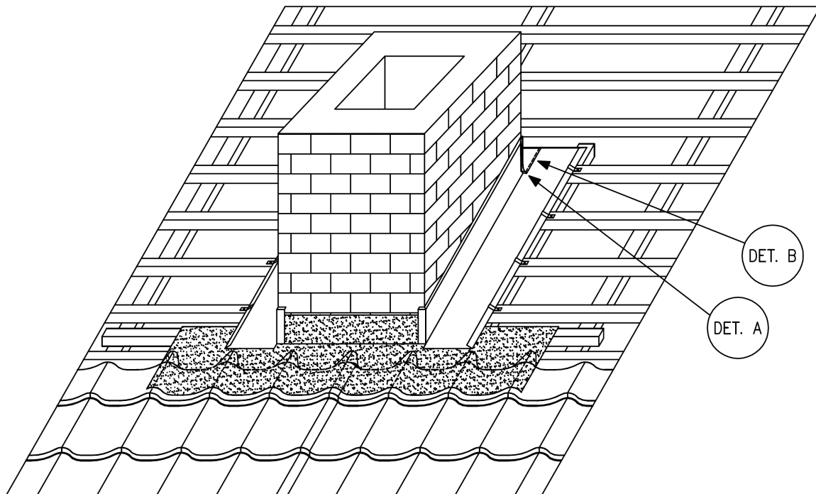
Obr. 17a: Osazení klempířských prvků
