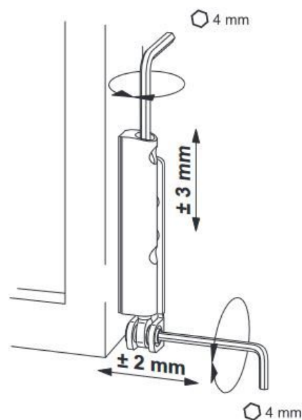
Obr. 70 – Schéma seřízení
