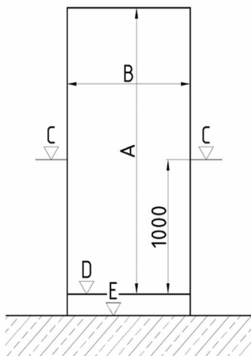
Obr. 15 – Zaměřené rozměry stavebního otvoru pro vstupní dveře
