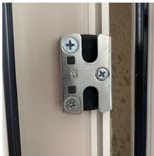
Obr. 79 – Bezpečnostní okenní uzávěr
