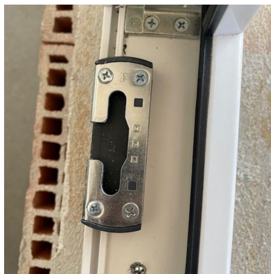
Obr. 81 – Výklopný bezpečnostní uzávěr – pouze v případě ventilace
