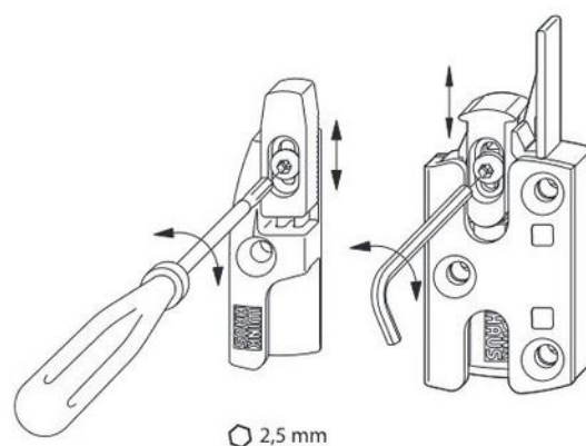
Obr 76 – Schéma posunu výšky protiplechu
