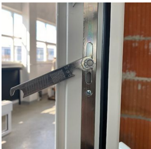
Obr. 73 – Seřízení přitlaku excentrickým čepem
