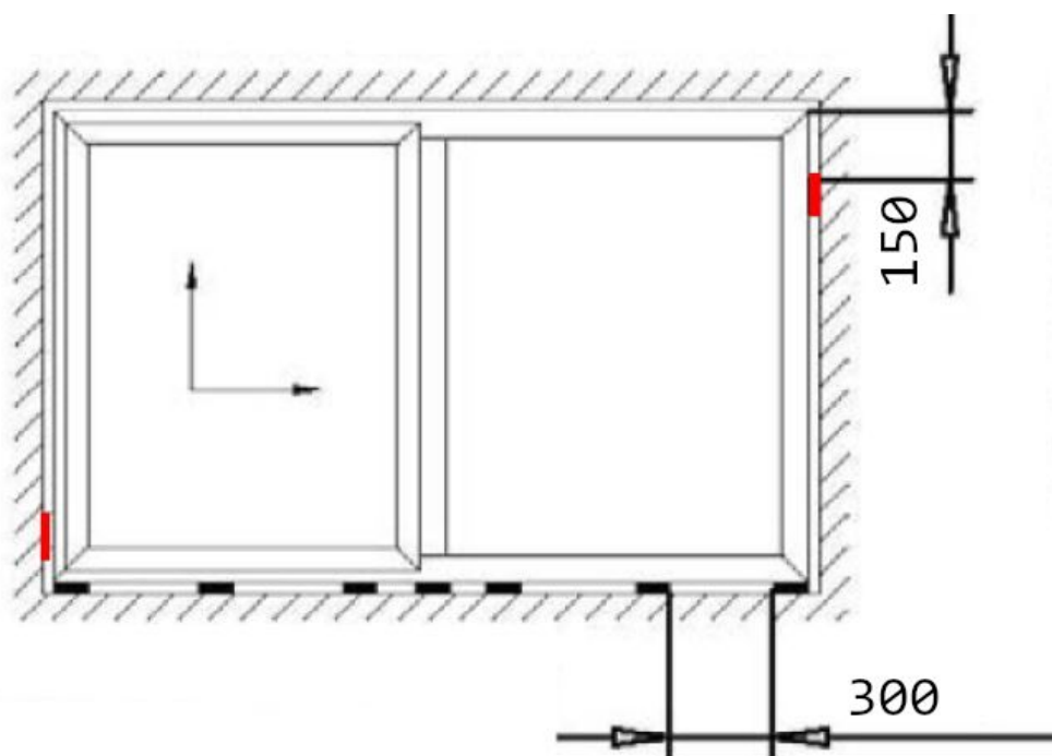
Obr. 63 – Doporučené rozmístění podložek pod HST
