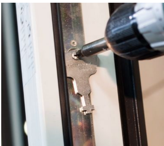
Obr. 55 – Pojistný klíč na křídle PSK systému
