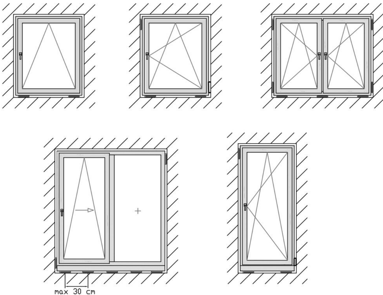
Obr. 31 – Doporučené rozmístění nosných a distančních podložek
