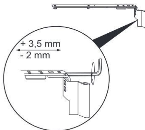
Obr. 72 – Schéma seřízení ventilačních nůžek
