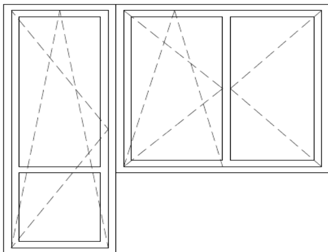
Obr. 11 – Schéma použití spojovacího profilu u balkonové sestavy
