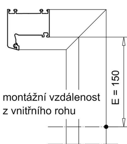
Obr. 33 – Vzdálenost kotvení od vnitřního rohu rámu
