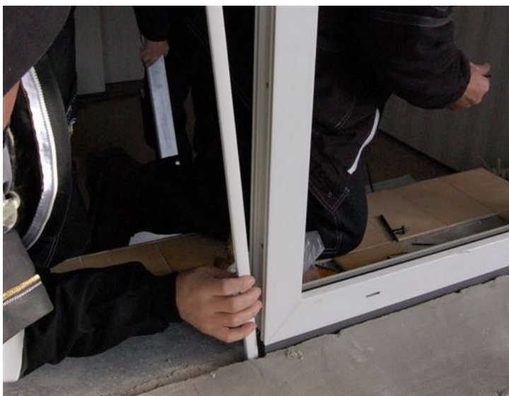
Obr. 13 – Vložení spojovacího profilu
