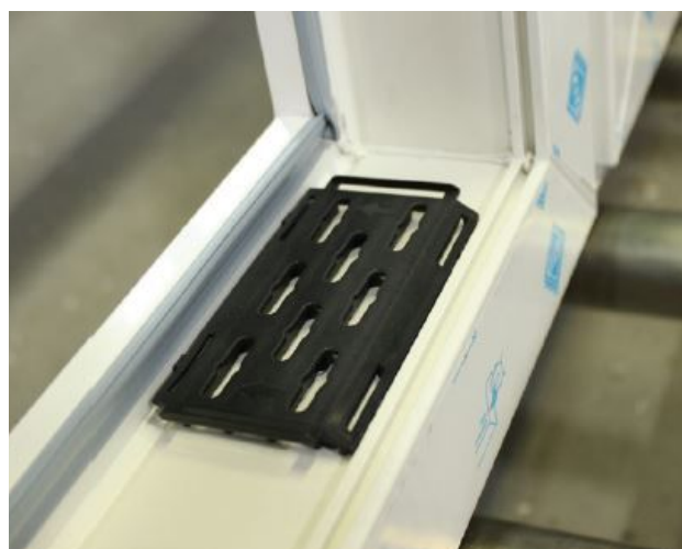
Obr. 95 – Distanční podložky
