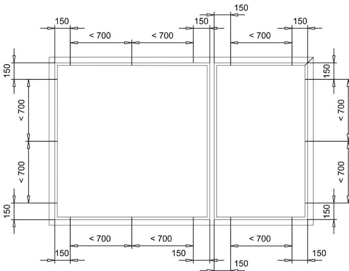
Obr. 32 – Doporučené rozteče kotevních prvků oken a portálů – kotevní plán
